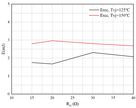
图 8. 开关损耗 二极管 Figure 8. Switching losses of Diode I_F=30\text{A} , V_{CE}=600\text{V}
