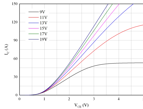
图 2. 典型输出特性 ( T_{vj}=150^{\circ}C )
