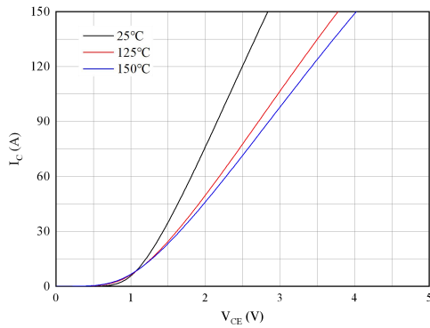
图 1. 典型输出特性 ( V_{GE}=15V )
