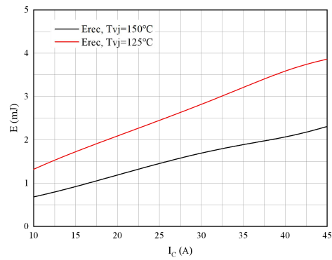
图 7. 开关损耗 二极管 Figure 7. Switching losses of Diode R_{Gon}=15\Omega , V_{CE}=600\text{V}
